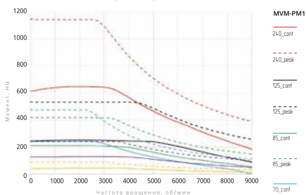
Мощностные характеристики
