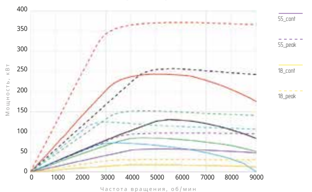
Мощностные характеристики
